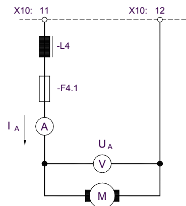
5-4 Q1-Motor-Mess-1
