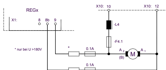
4-12 Q1-Ankerspannungsregelung-1
