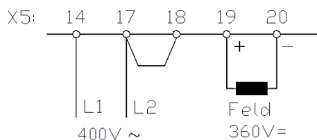
4-7 Q1-Q2-Feld400-360-1
