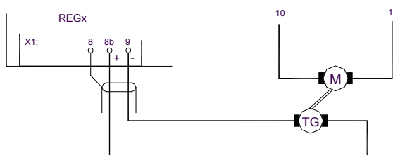
4-11 Q1-Tachoregelung-1
