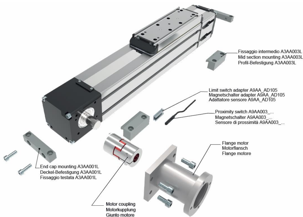
Abbildung 4: Zubehör MTB105
