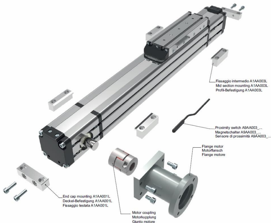
Abbildung 2: Zubehör MTB55
