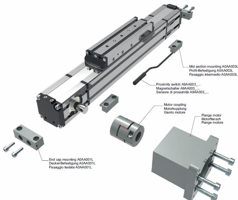
Abbildung 1: Zubehör MTB42
