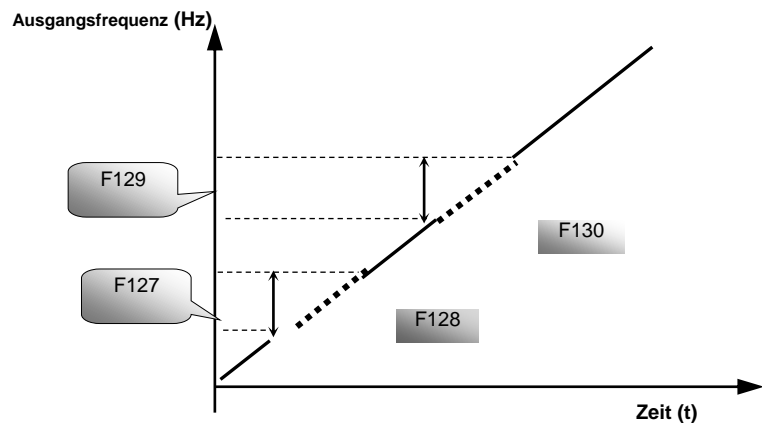
Abbildung 9-2 Ausblendfrequenz
