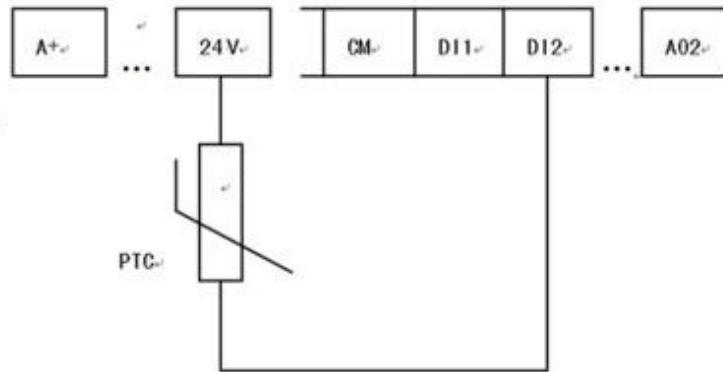
Abbildung 9-6 PTC-Überhitzungsschutz
