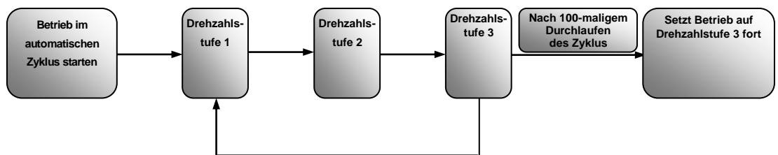
Abbildung 9-10 Automatischer Zyklusbetrieb
