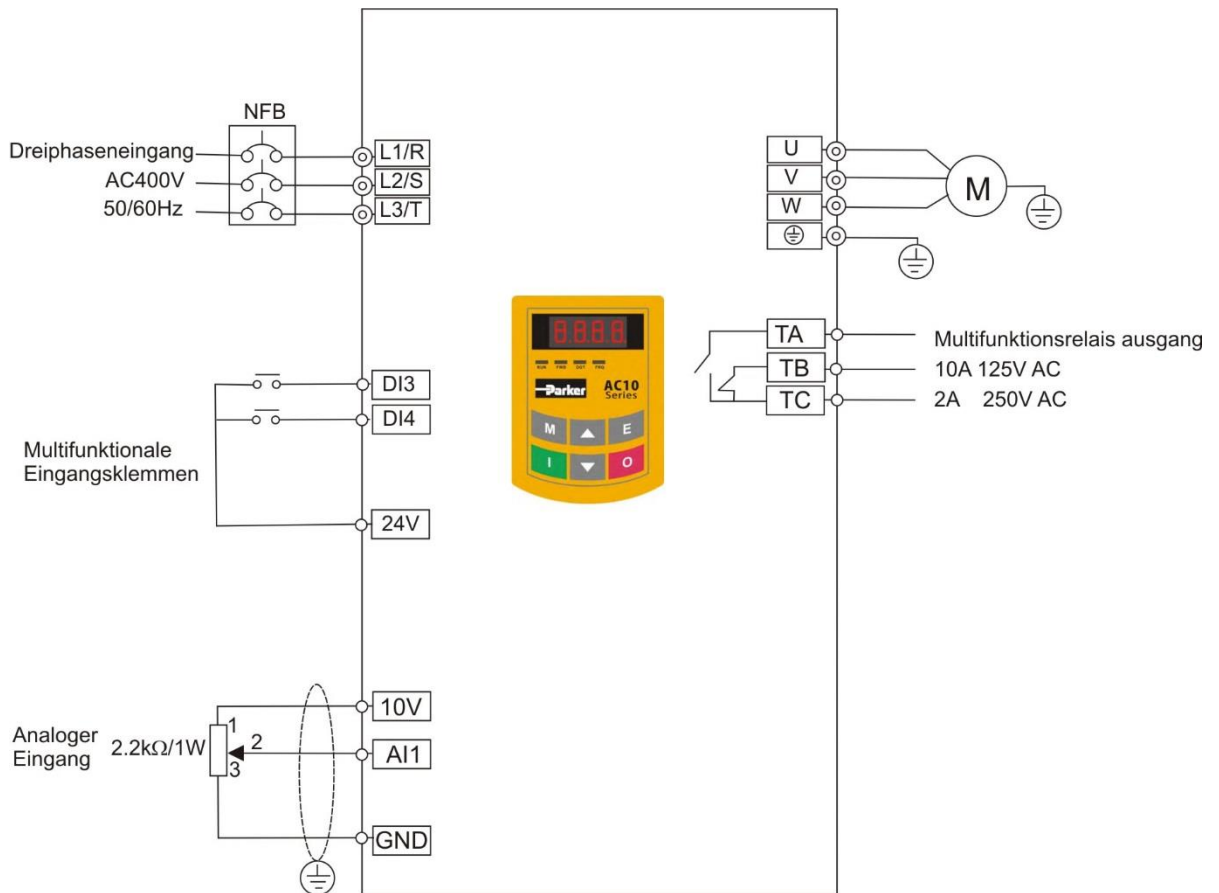
Abbildung 8-3 Schaltplan 3
