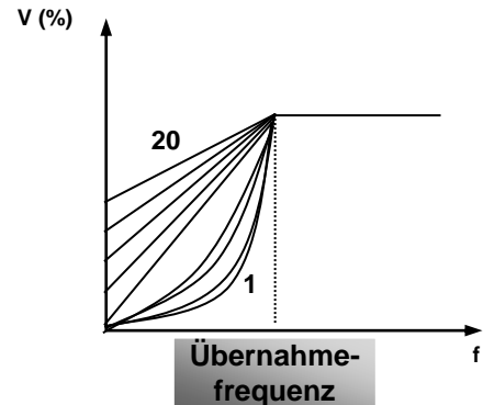
Abbildung 9-3 Drehmomenterhöhung
